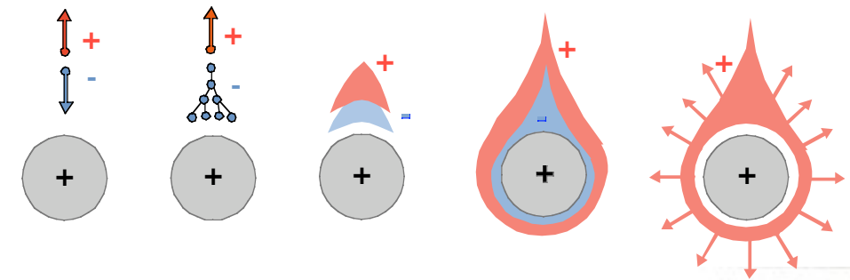
Fig. 6.1.1 ionization
